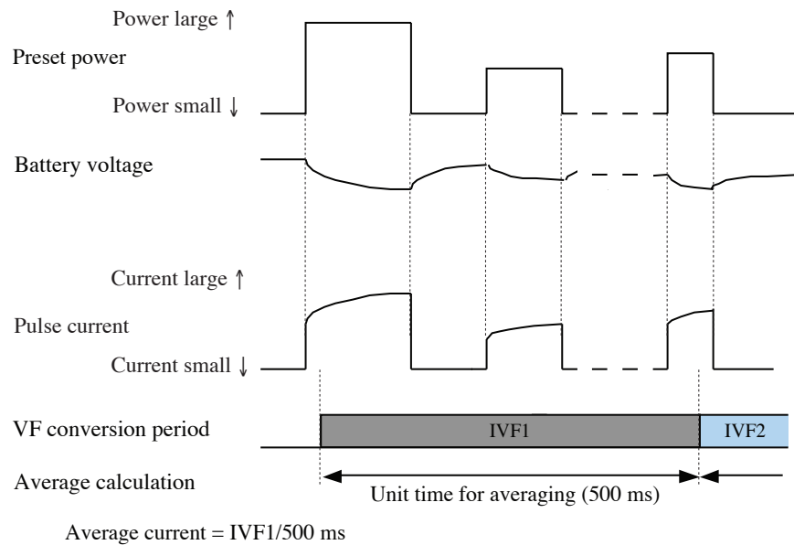
Fig. A-12 CP Pulse Discharge Example
